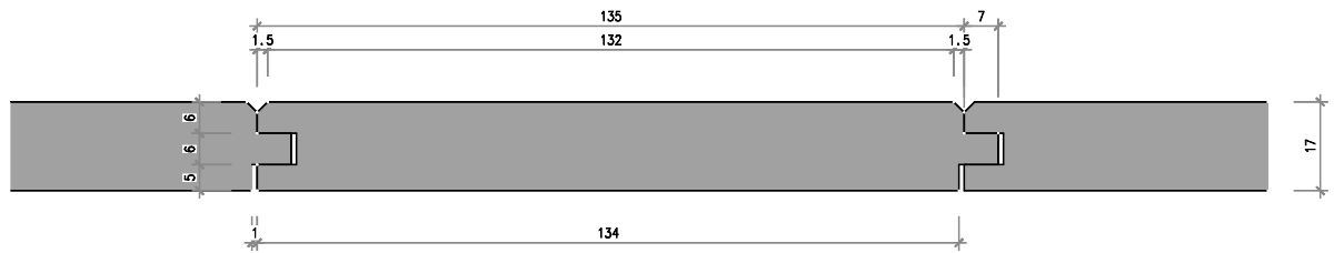
Nr. 1103-2k-01 Fastäfer 17/135 mm, Fase 1.5 mm
