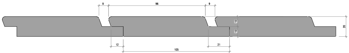
Nr. 6001-09-03 Wechselfalz mit Rhomboid 20°
