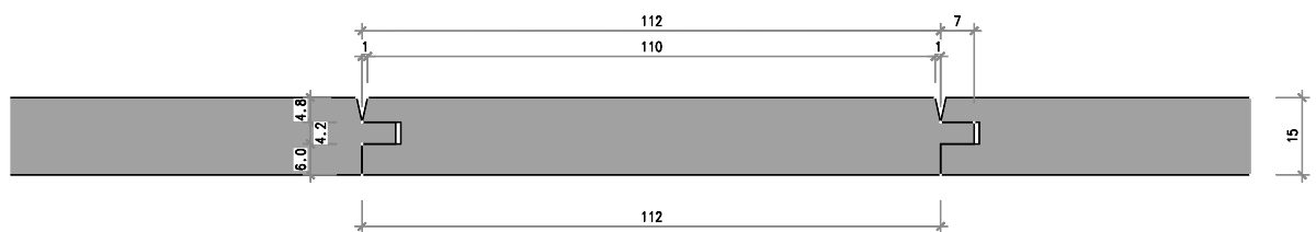
Nr. 1205-02-00 Steilfastäfer 15/112 mm
