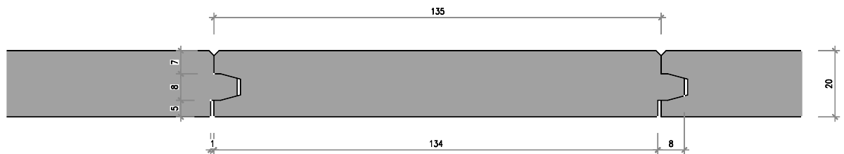
Nr. 4663-M2k-01 Spitzkamm 20/135 mm, Fase 1.5 mm
