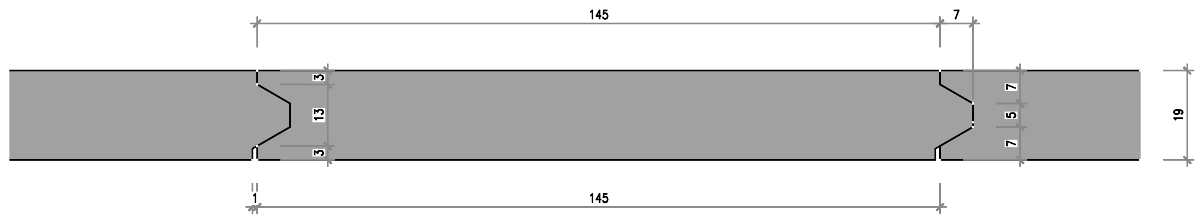
Nr. 4665-L Blindschalung 19/145 mm, Kamm 30°
