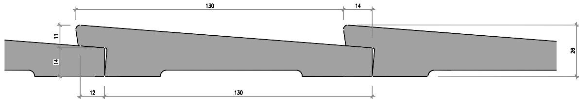
Nr. 7601-00-03 Stülpschalung Falz 14/26/130 mm, Rückseitig ausgekehlt
