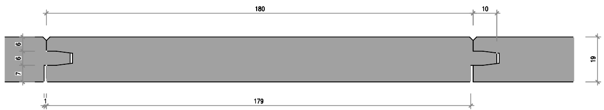
Nr. 4153-2k-01 Spezial Fastäfer 19/180 mm, Fase 1.5 mm
