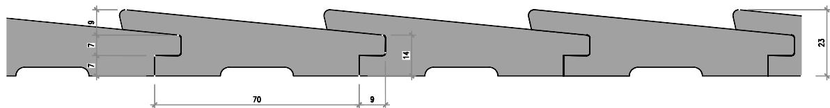
Nr. 7702-00-03 Stülpschalung N+K 14/23/70 mm, Rückseitig ausgekehlt
