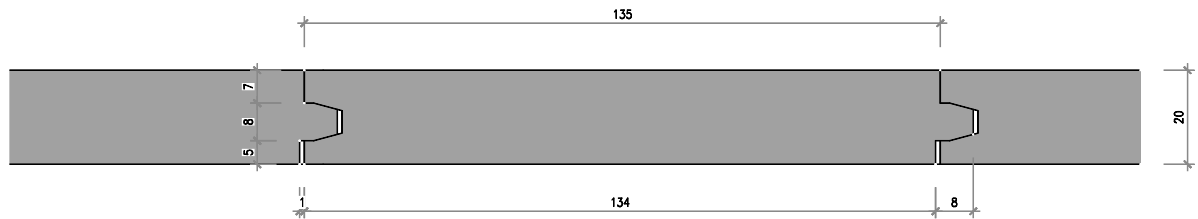
Nr. 4665-M Spitzkamm 20/135 mm
